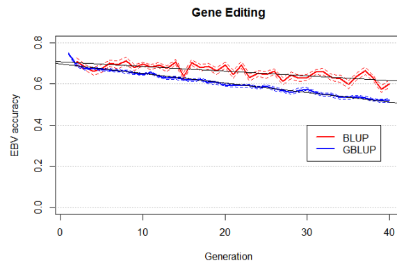
Figura 3. Precisión de las evaluaciones genéticas a lo largo de las generaciones de selección para GBLUP y BLUP en un programa tradicional o de edición genética (error estándar de las 25 réplicas en línea discontinua)
